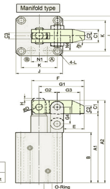
油路板式:
