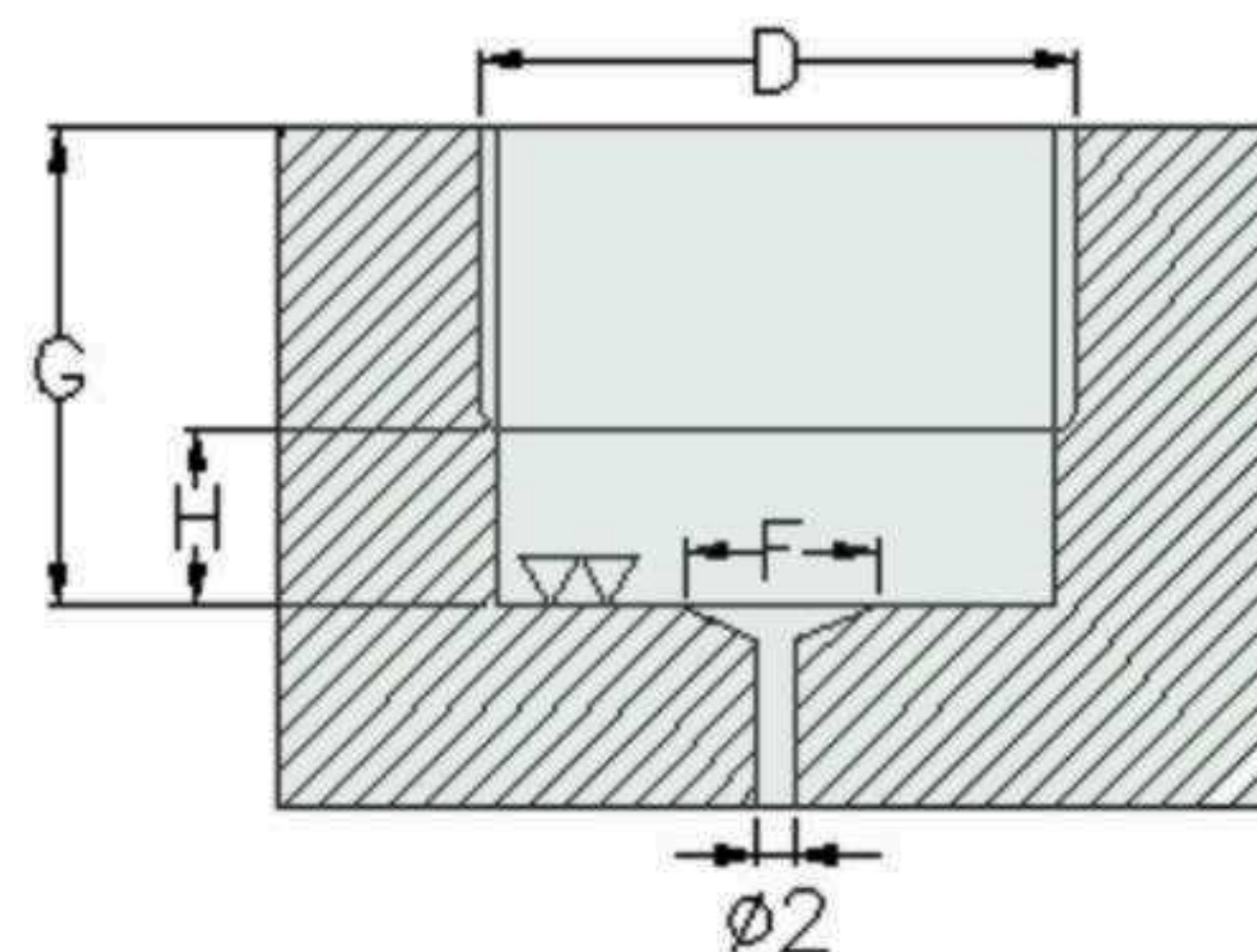
安裝尺寸 Mounting Diagram
