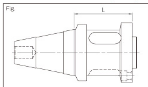
Hシャンク互換表 H Shank Compatibility Table
