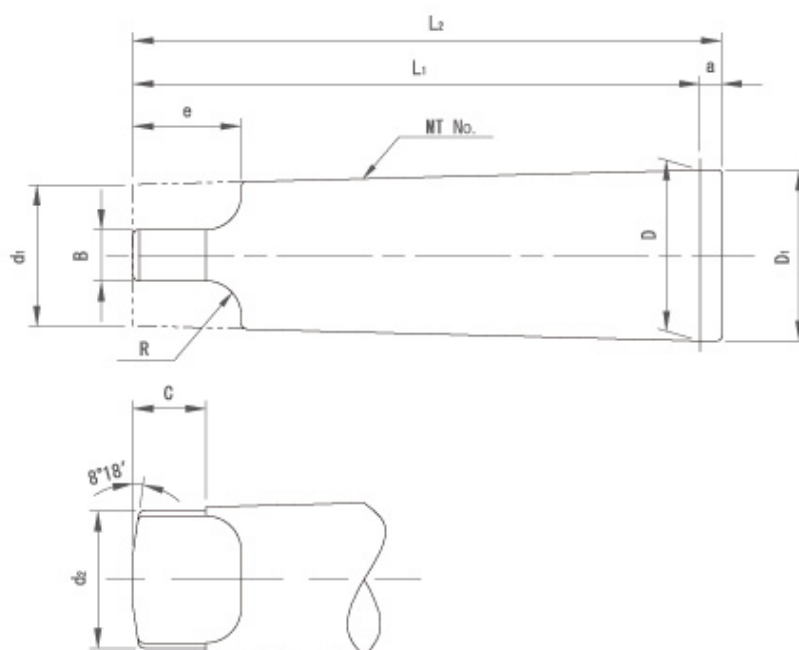
MT寸法表(タング式) MT Dimension Table(Tongue Type)
