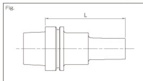
HSKシャンク互換表 HSK Shank Compatibility Table
