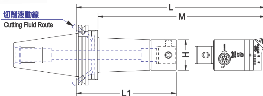
DIN69871B 搪孔刀柄 DIN69871B Taper Shank
