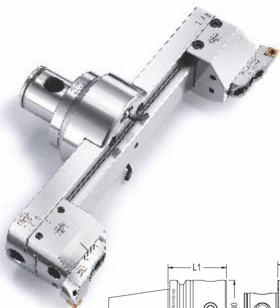
H100 系列-搪孔刀柄 Taper Shank
